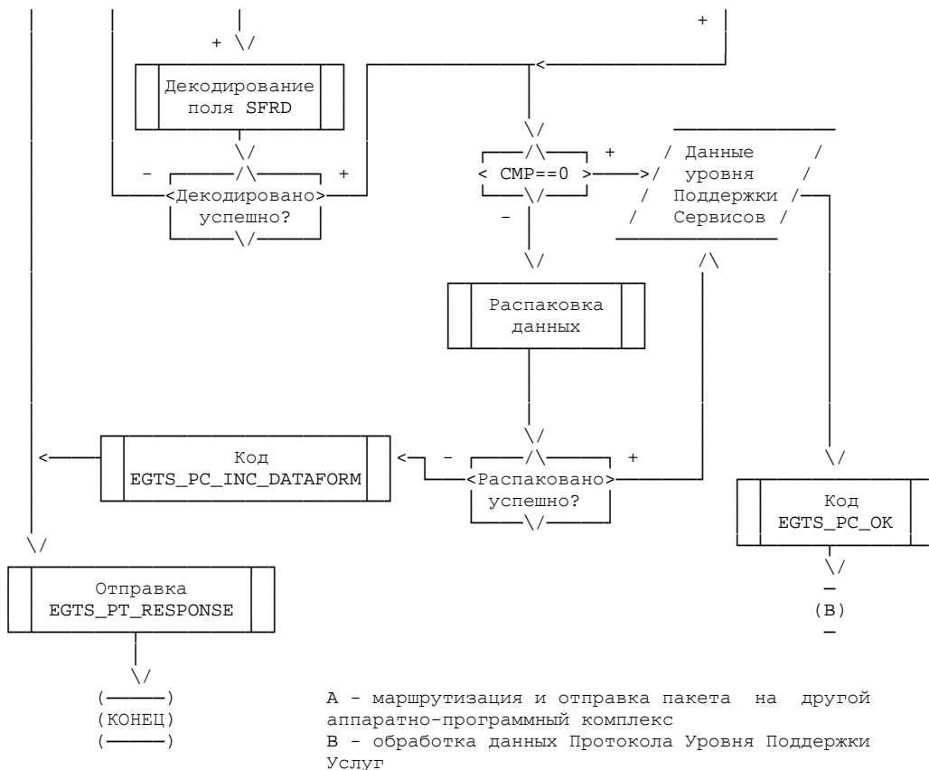
Рисунок 2. Блок-схема алгоритма обработки пакета данных протокола Транспортного уровня при приеме
